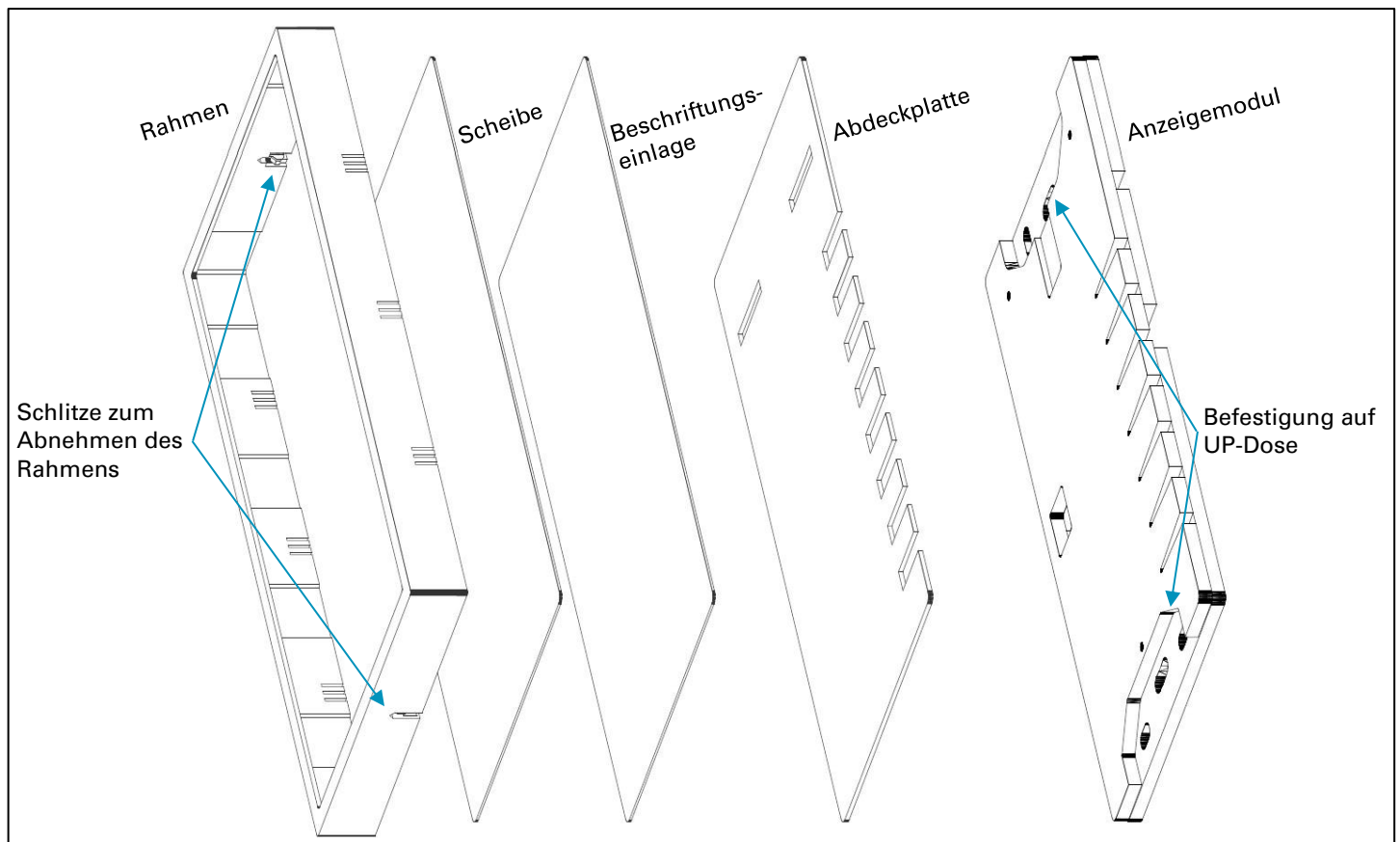
Bild 2: Explosionszeichnung
