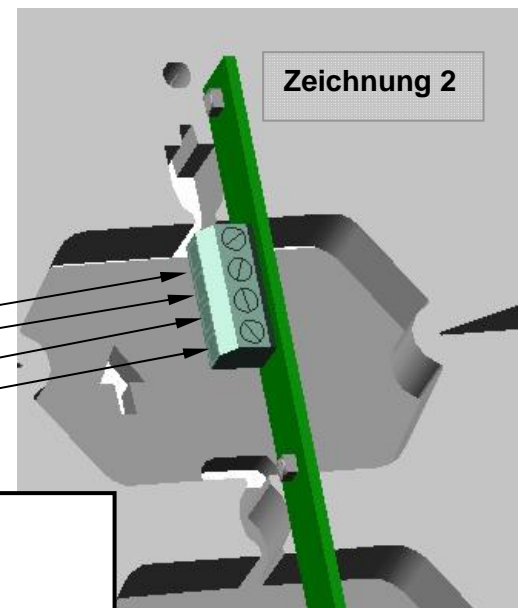
Anschaltbelegung LED-Platine
